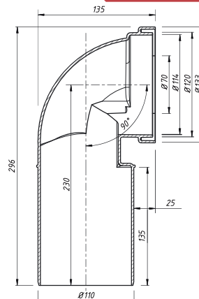
Труба фановая прямая 110 x 90
