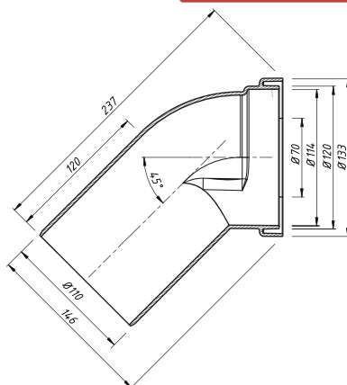
Труба фановая прямая 110 x 45
