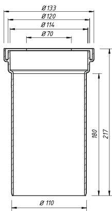
Труба фановая прямая 110
